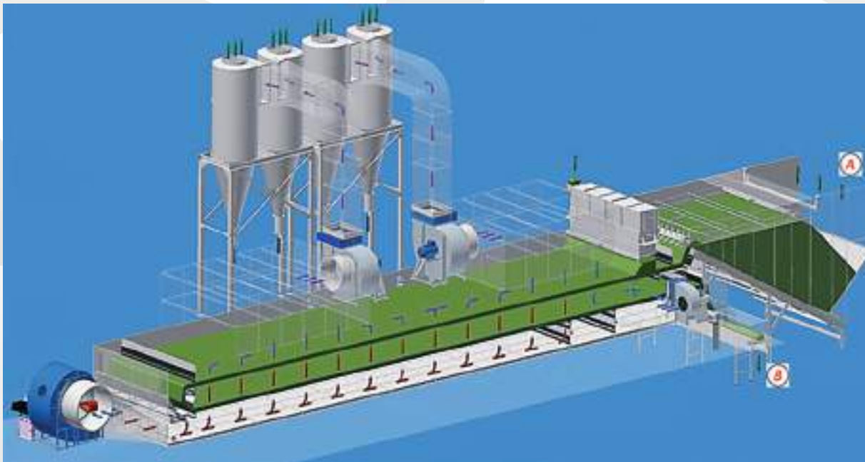
A Entrata prodotto umido / Moisture material entrance B Uscita prodotto secco / Dried material exit ■ Aria ambiente / Room air ■ Aria essiccazione / Drying air ■ Aria satura / Saturated air ■ Aria depurata / Clean air ■ Recupero polveri / Powder recovery
